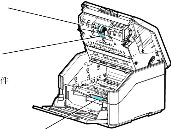
反轉輪組件
